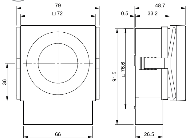
Tipo 12.71 Borne de jaula
