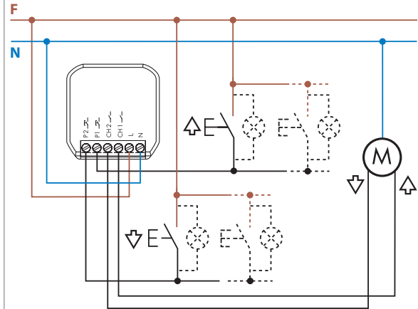
Tipo 13.S2 Conexión a 4 hilos
