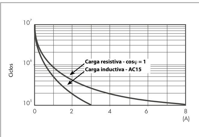
F 40.4 - Vida útil eléctrica (AC) en función de la carga
