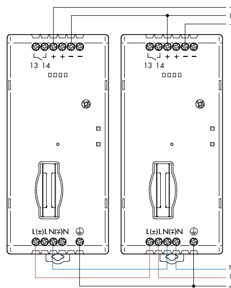
Conexión en serie
