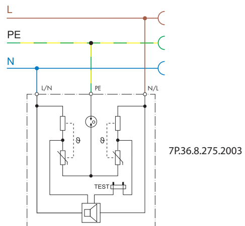
TT o TN-S MONOFÁSICA INCORPORADO EN EL ENCHUFE
