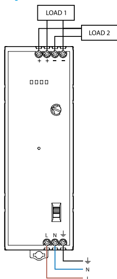
Esquema de conexión para el tipo 78.2A
