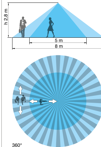
18.31...0031 - Instalaciones en techos altos
