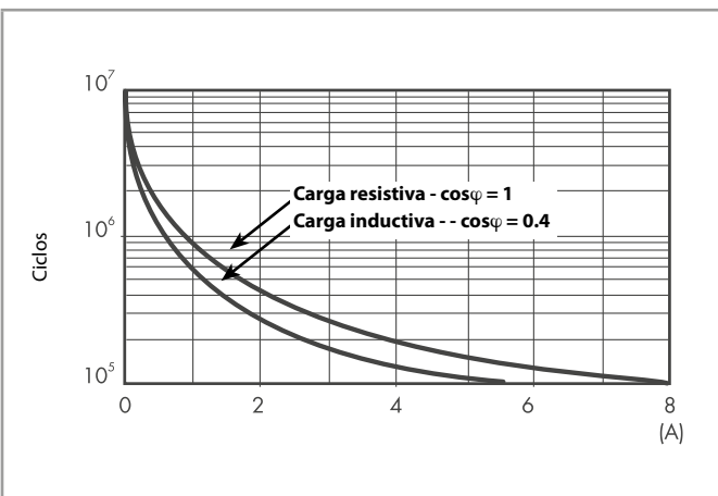
F 40.6 - Vida útil eléctrica (AC) en función de la carga
