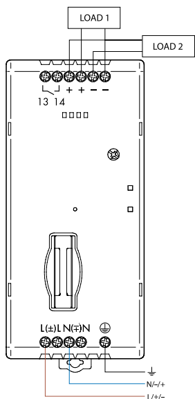
Conexiones básicas
