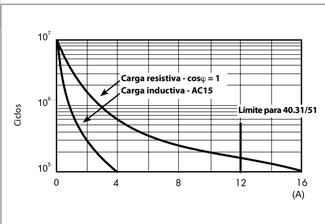
F 40.3 - Vida útil eléctrica (AC) en función de la carga
