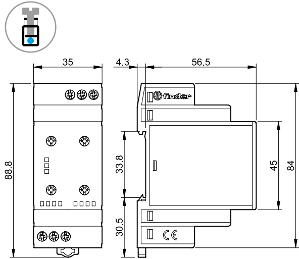
Tipo 70.31 Borne de jaula
