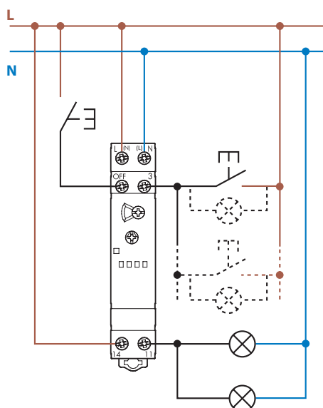
Conexión a 4 hilos
