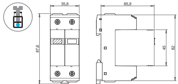
Tipo 7P.22 / 7P.27 / 7P.42 Borne de jaula
