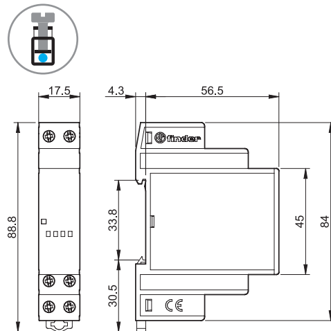
Tipo 13.81 Borne de jaula
