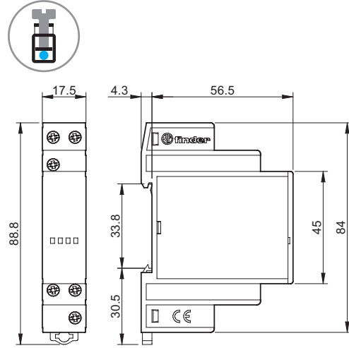
Tipo 13.31/13.91 Borne de jaula
