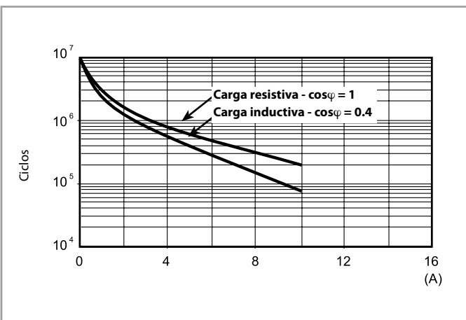
F 40.5 - Vida útil eléctrica (AC) en función de la carga
