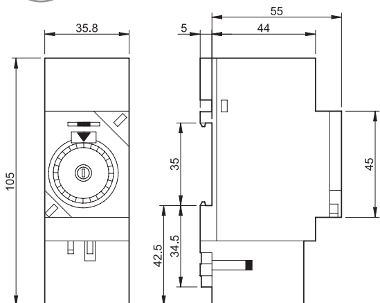
Tipo 12.31 Borne de jaula
