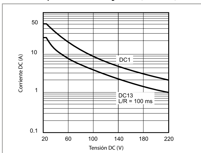
H 67 - Máximo poder de corte con cargas en DC (67.xx-x500)
