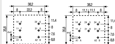
62.22-0300 Vista parte inferior 62.23-0300 Vista parte inferior
