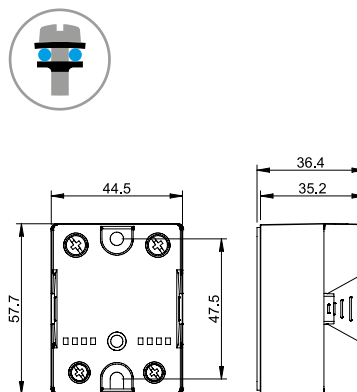
Tipo 77.x5 Bornes a pletina
